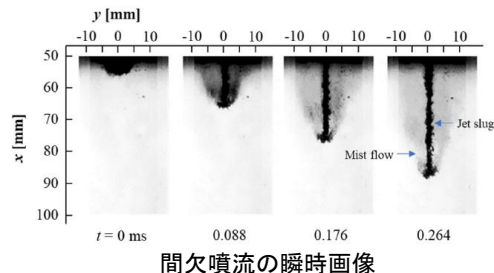
間欠噴流の瞬時画像
