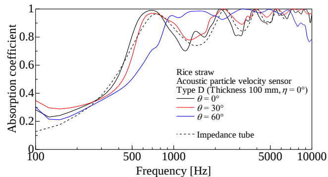
稲藁の吸音率(軽めのグラスウールに匹敵する特性を持つ)
