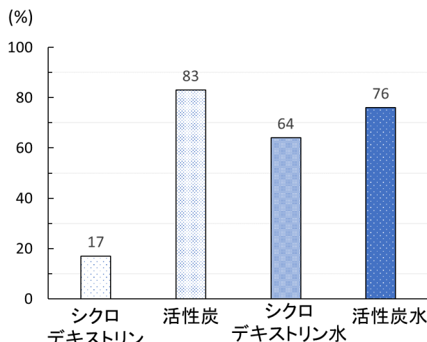
図1. シクロデキストリンおよび活性炭によるアセトンの消臭効果
