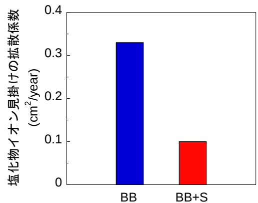
高炉セメントB種(BB)にシリカフューム(S)を加えた3成分系結合材コンクリートの塩分浸透抵抗性
