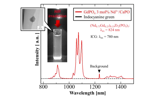
図 Nd 3+ -NASICON蛍光体のTEM画像と発光写真と発光スペクトル
