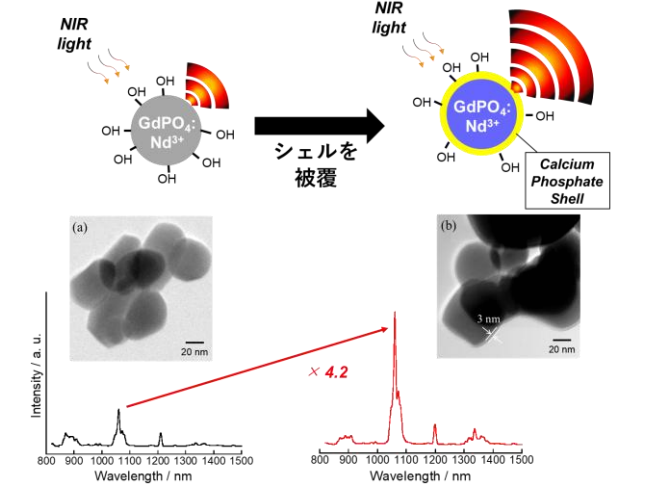
図 GdPO 4 : 3 mol% Nd 3+ コアとGdPO 4 : 3 mol% Nd 3+ /CaPOコアシェル蛍光体のTEM画像と発光スペクトル
