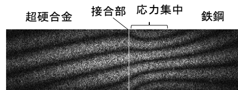
材料変形可視化のためのスペックルパターン干渉計
