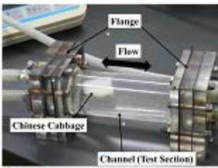
交番流式洗浄装置（野菜洗浄の例）
