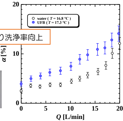
洗浄率に対するポンプ流量の関係（UFBの洗浄効果）
