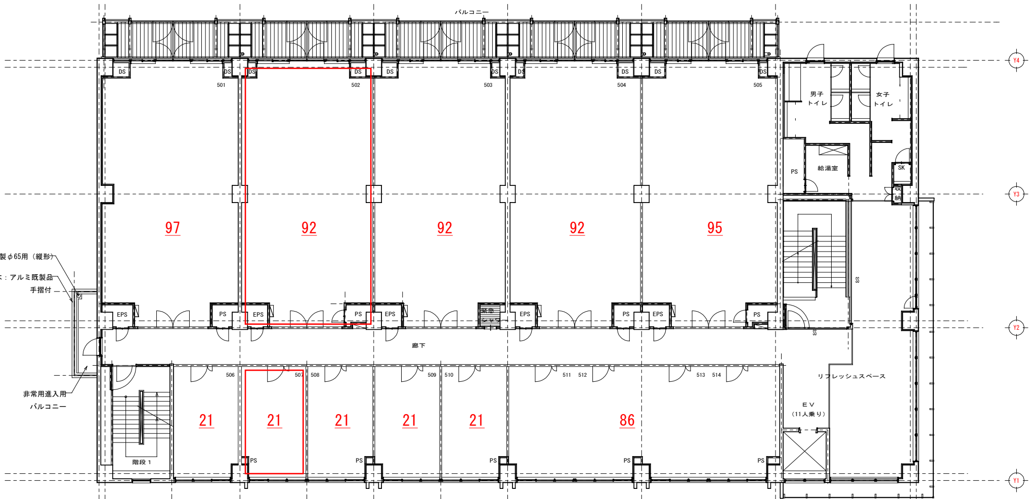
5階平面図
