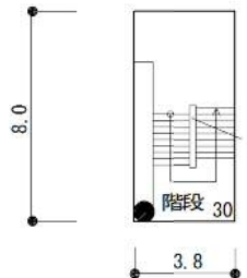
R階平面図 S = 1 : 300 30㎡
