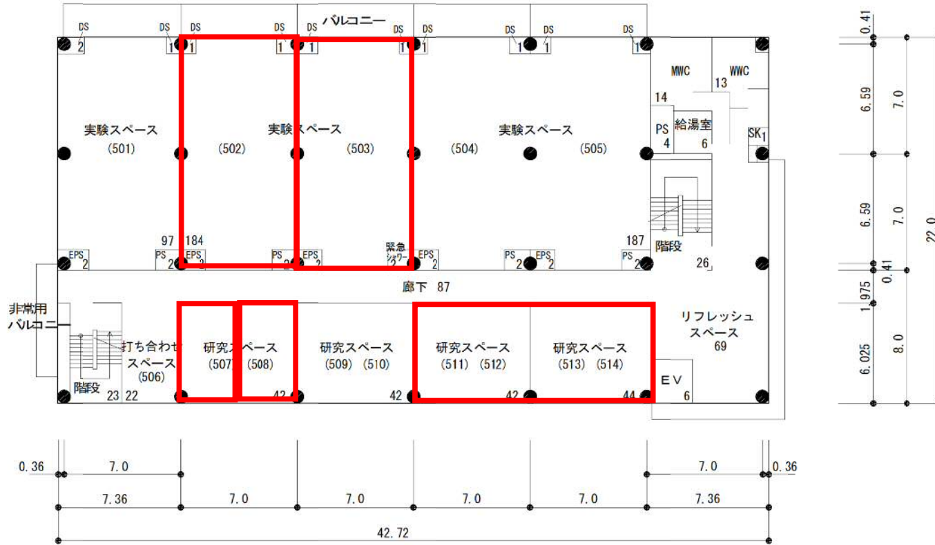
5階平面図 S = 1 : 300 940㎡
