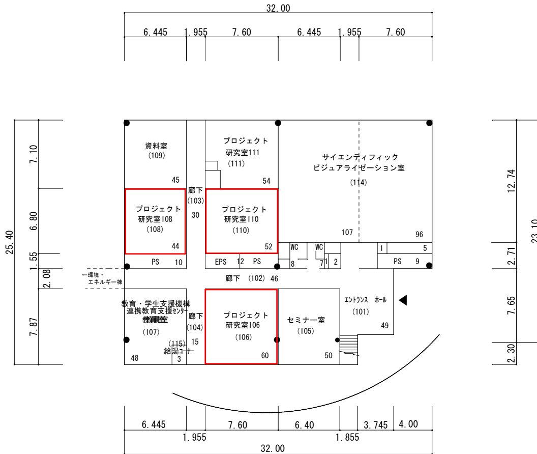
1階平面図 754m 2
