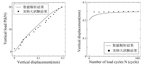
単調载荷過程・繰り返し载荷過程における解析結果
