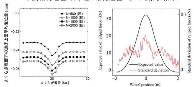
レール継目での道床上面変位分布
