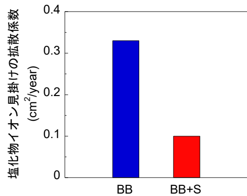
高炉セメントB種(BB)にシリカフェーム(S)を加えた3成分系結合材コンクリートの塩分浸透抵抗性
