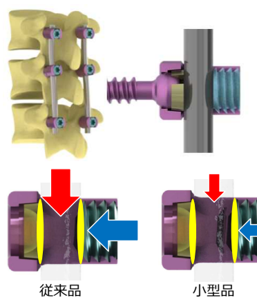
図1 高摩擦係数表面による小型化の例
