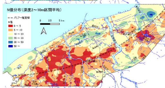
新潟市表層の土質とN値の推定例（深度 2～10m平均）
