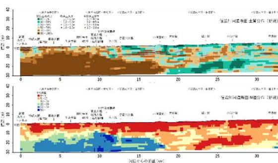
信濃川下流の河道沿いの推定地盤断面(土質・N値)
