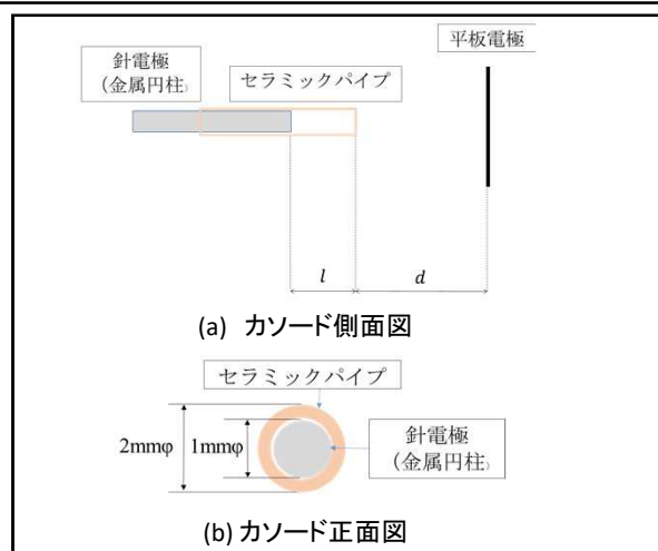
図1 セラミック被覆カソードの概略図
