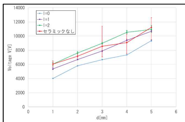
図2 放電開始電圧特性
