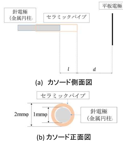
図1 セラミック被覆カソードの概略図
