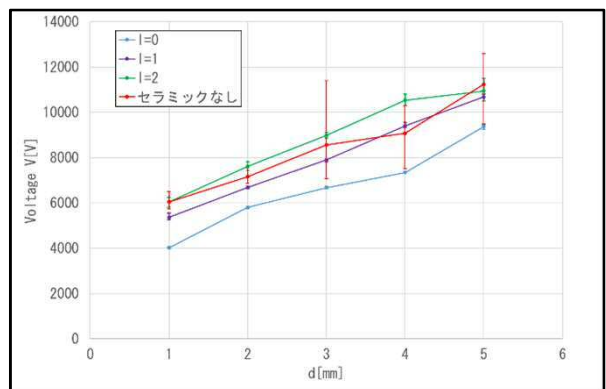
図2 放電開始電圧特性
