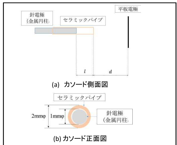
図1 セラミック被覆カソードの概略図
