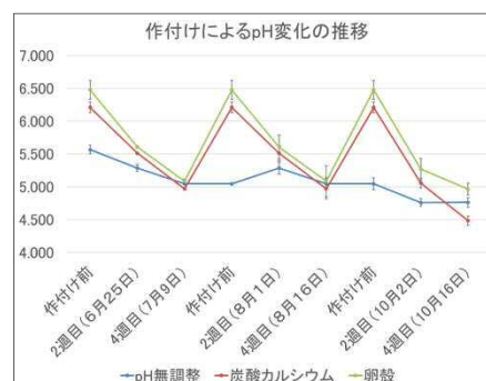
土壌に添加した場合の中和効果
