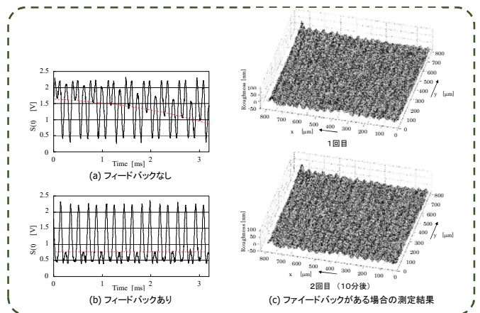
図2 表面形状測定結果
