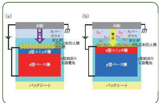
(a) 電荷蓄積型および(b) 元素侵入型PIDのメカニズム
